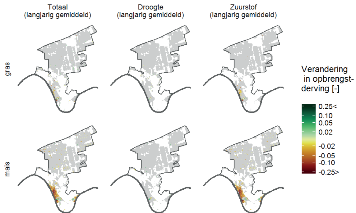
FIGUUR 7.13 VERANDERINGEN IN OPBRENGSTDerving (TOTAAL: LINKS; DROOGTESTRESS: MIDDEN; ZUURSTOFSTRESS: RECHTS) VOOR GRAS (BOVENSTE RIJ) EN MAIS (ONDERSTE RIJ) IN DEELGEBIED STEGEREN ALS GEVOLG VAN EEN INRICHTINGSMaatregel TEN OPZICHT VAN DE HUIDIGE SITUATIE MET IN HET GROEN EEN VERBETERING EN IN HET ROOD EEN VERSLECHTERING ALS GEVOLG VAN DE MAATREGEL ZOALS BEREKEND MET WATERWIJZER LANDBOUW (WWL-TABEL)
