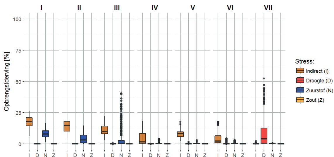
FIGUUR 6.3 SPECIFICATIE VAN OPBRENGSTDerving IN AANDEEL INDIRECTE EFFECTEN (I) EN DIRECTE EFFECTEN (MET DROOGTE- (D), ZUURSTOF- (N) EN ZOUTSTRESS (Z)) WEERGEGEVEN MET BOXPLOTS PER GRONDWATERTRAP VOOR HET GEWAS ZETMEEL- EN CONSUMPTIEAARDAPPEL VOOR ALLE WEERJAREN IN DE PERIODE 1981 - 2010
