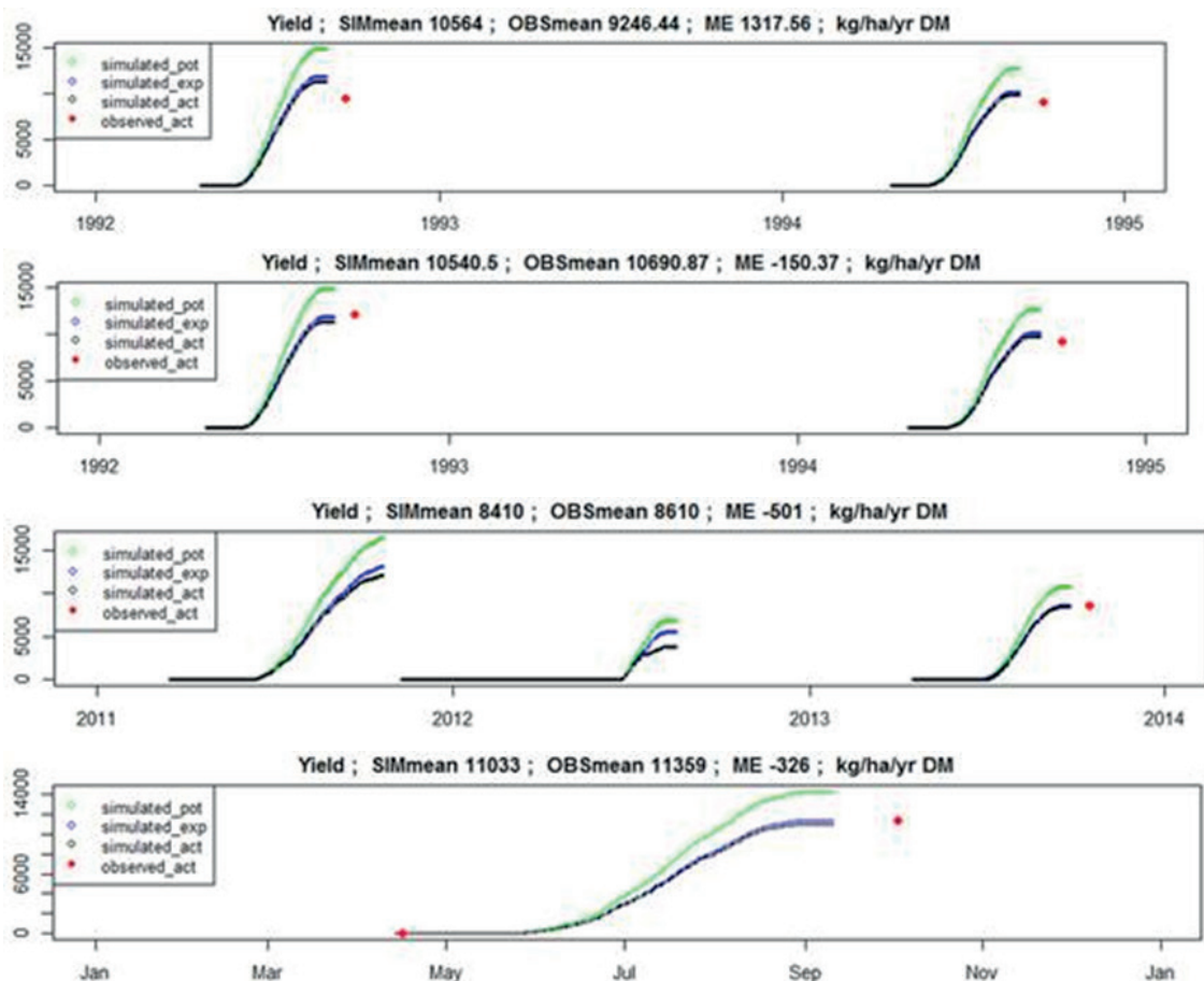
FIGUUR 7.3 MODELRESULTATEN EN METINGEN VAN GEWASOPBRENGSTEN VOOR AARDAPPEL, VAN BOVEN NAAR BENEDEN: G) BORGERSWOLD3, H) BORGERSWOLD13, I) RUSTHÖVEB7, J) VREDEPEEL26. GROEN: BEREKENDE POTENTIËLE OPBRENGST, BLAUW: DE BEREKENDE EXPLOITEERBARE OPBRENGST, ZWART: DE BEREKENDE ACTUELE OPBRENGST, ROOD: DE GEMETEN OPBRENGST
