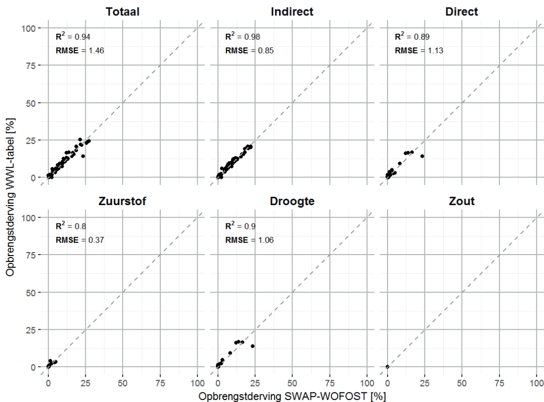
FIGUUR 6.4 VERGELIJKING VAN OPBRENGSTDerving BEREKEND MET SWAP-WOFOST (HORIZONTALE AS) VERSUS DE WWL-TABEL (VERTICALE AS), VOOR HET GEWAS ZETMEEL- EN CONSUMPTIEAARDAPPEL, BOFEK 304, METEOGEGEVENS VAN DE KOOP VOOR HET JAAR 1981. DE STIPPELIJN IS DE 1:1 LIJN. HOE DICHTER DE PUNTEN BIJ DEZE LIJN LIGGEN, DES TE BETER KOMEN DE BEREKENINGEN MET SWAP-WOFOST EN DE METARELATIES OVEREEN
